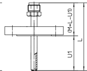
model 2 F/3F DIN-flange DN50/PN10/40 model B1 (DIN EN 1092-1) DN25/PN10/40 model B1 (DIN EN 1092-1)
